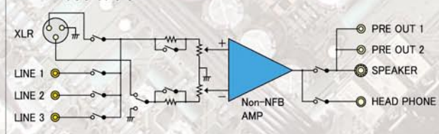
sa1.0 ブロックダイアグラム
